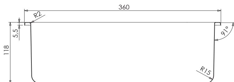
SEZIONE A-A
