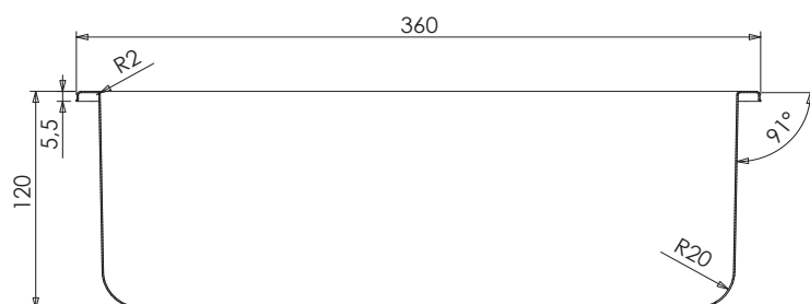
SEZIONE A-A
