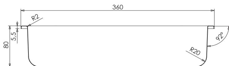
SEZIONE A-A
