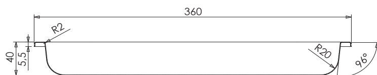
SEZIONE A-A
